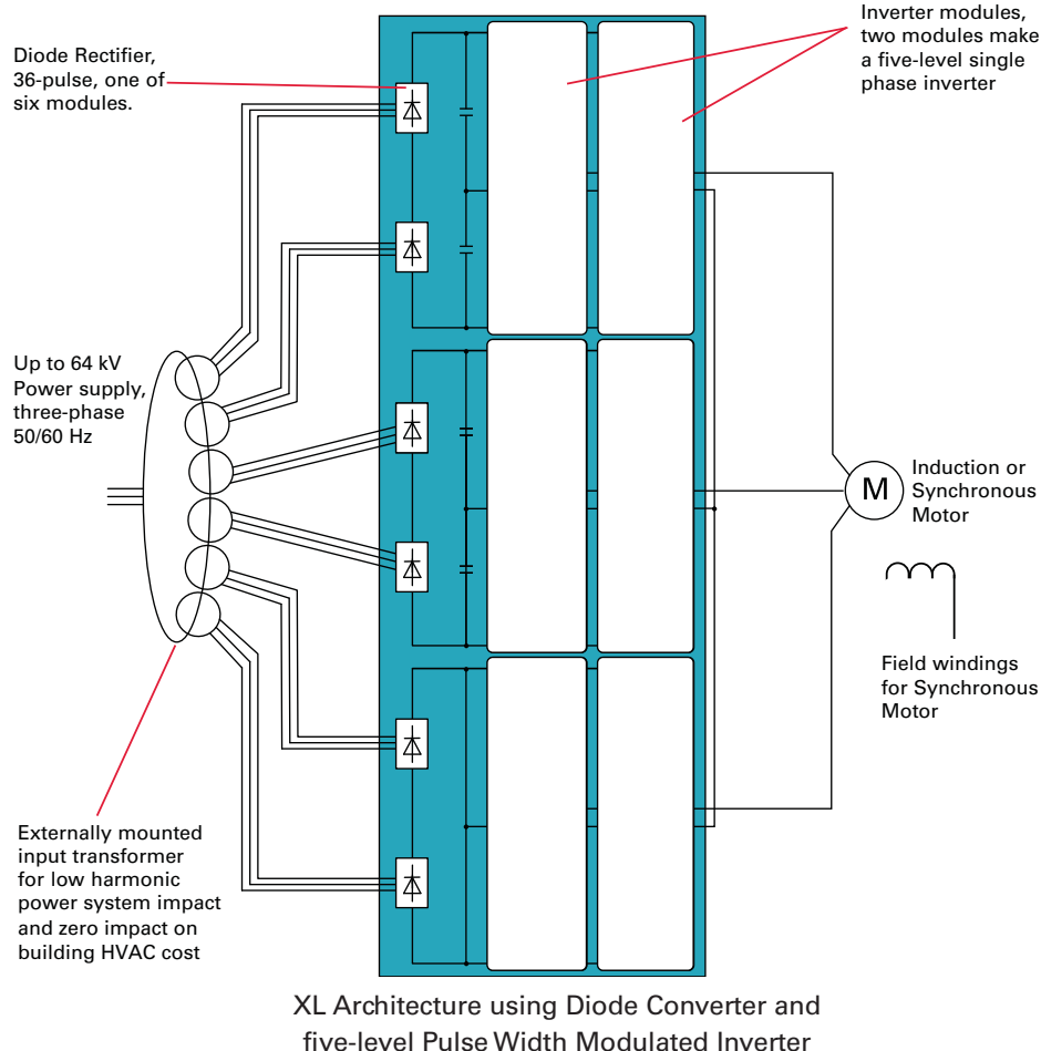
20 MVA VFD Power Module
