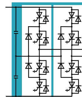
15/30 MVA Power Module
