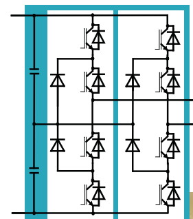
20 MVA VFD Power Module
