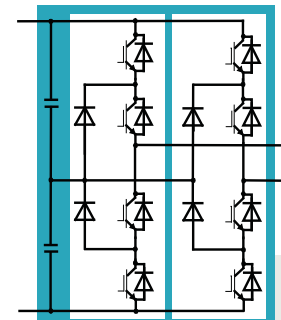
8 MVA VFD Power Module
